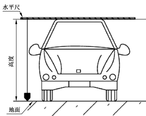
图 B.3 车辆高度的测量示意
