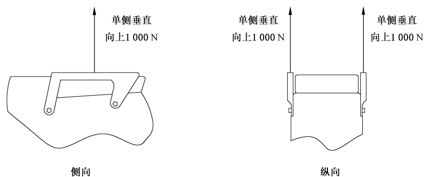
图 B.2 双手柄装置拉力试验示意图
