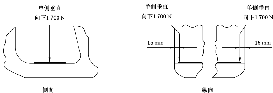
图 C.2 踏板压力试验示意图
