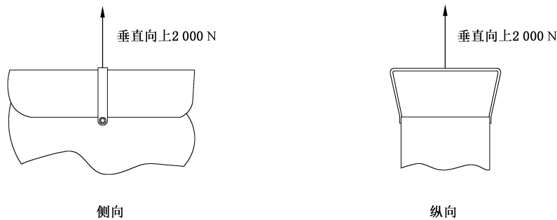
图 A.1 拉带装置拉力试验示意图
