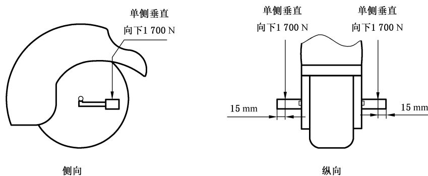
图 C.1 脚踏压力试验示意图
