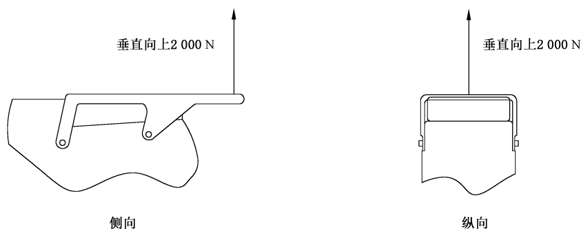
图 B.1 单手柄装置拉力试验示意图
