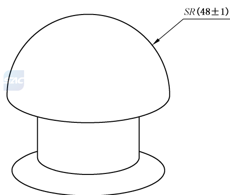
图 17 半球砧
