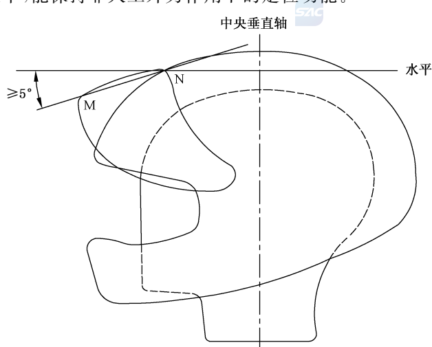
图 4 护目镜打开位置
