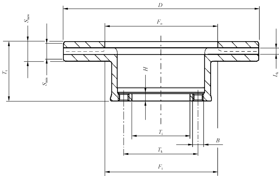
图 G.3 壶型
