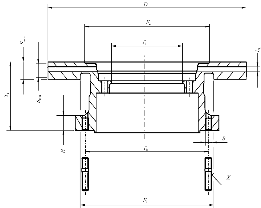
图 G.5 双凸缘型
