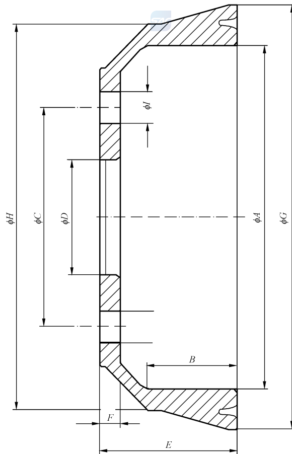
图 G.6 制动鼓
